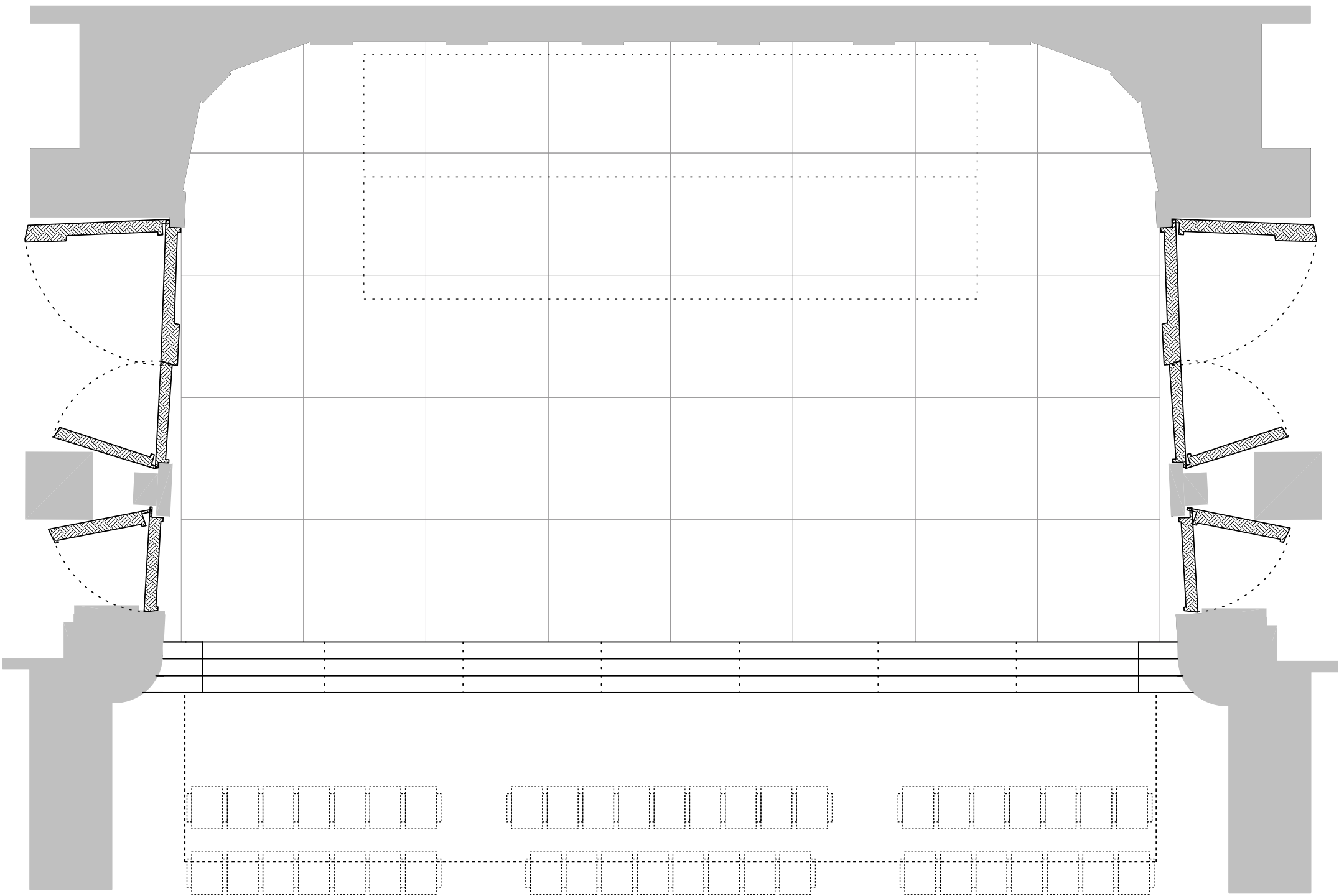
三井住友海上しらかわホール舞台平面図 (1マス:1間×1間)
